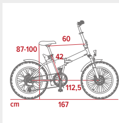
Dimensioni e-bike
