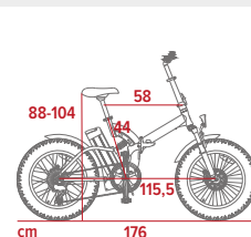
Dimensioni e-bike
